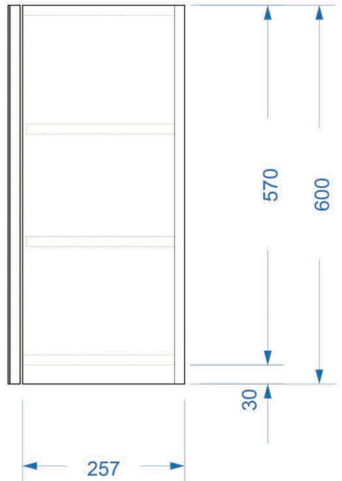
boční pohled
